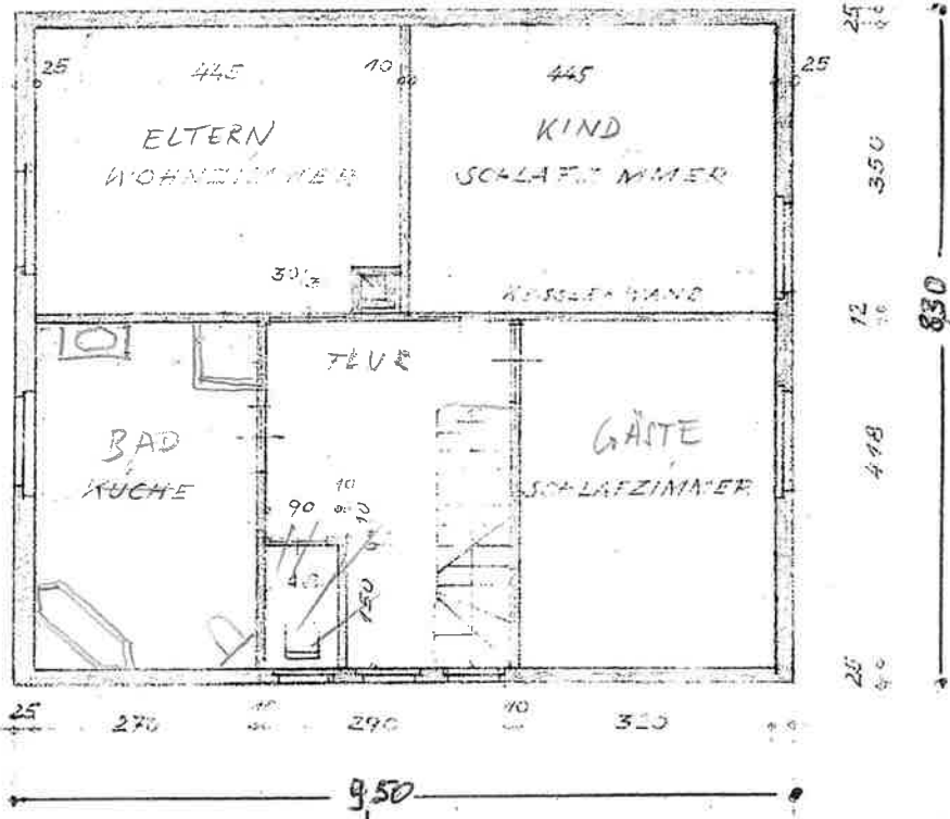
1. OBERGESCHOSS
