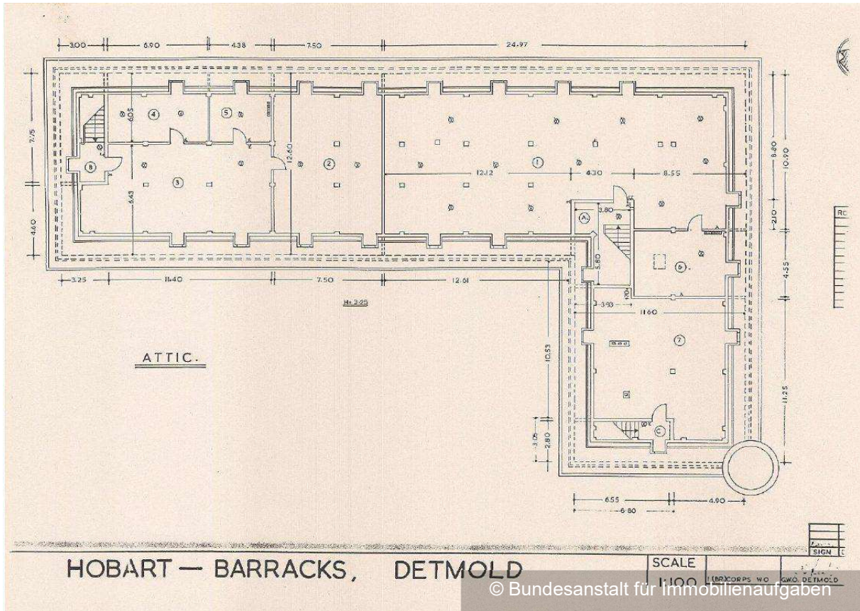
Grundriss Dachgeschoss
