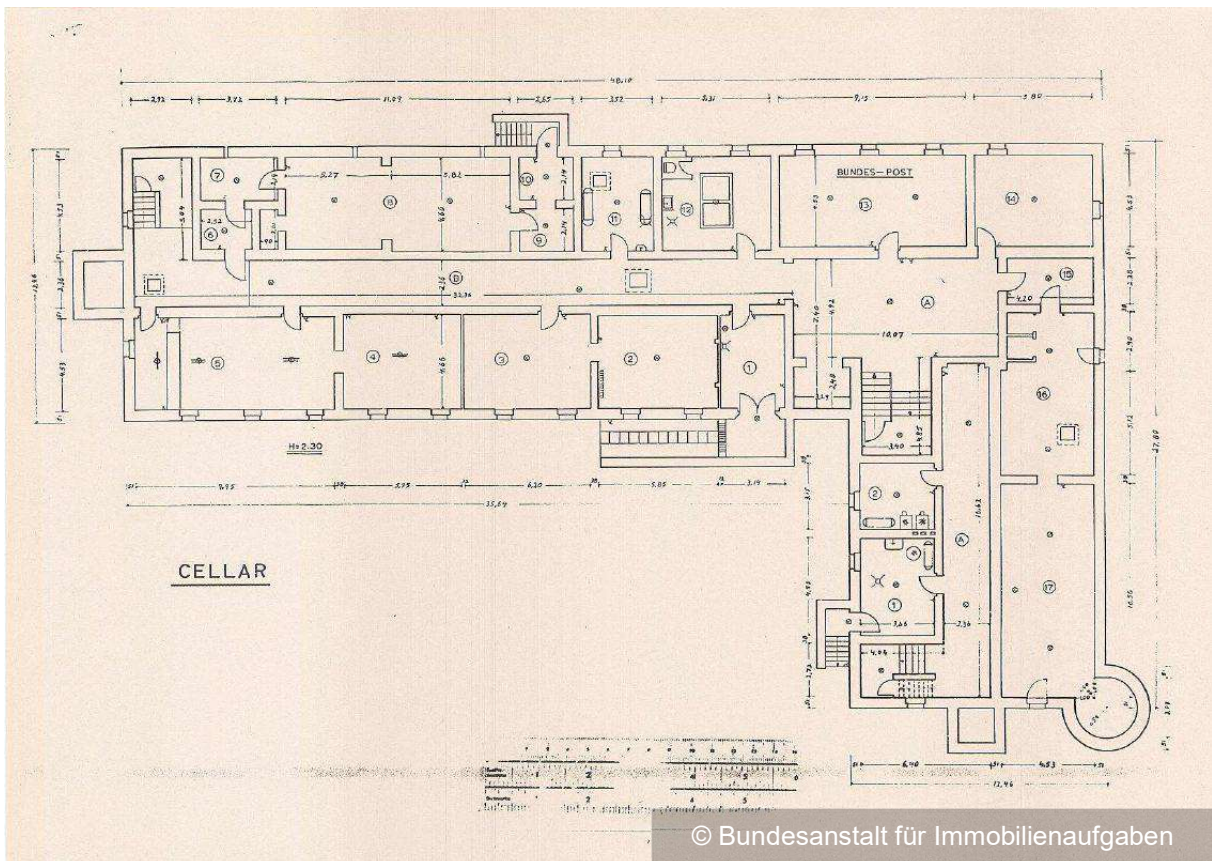
Grundriss Kellergeschoss
