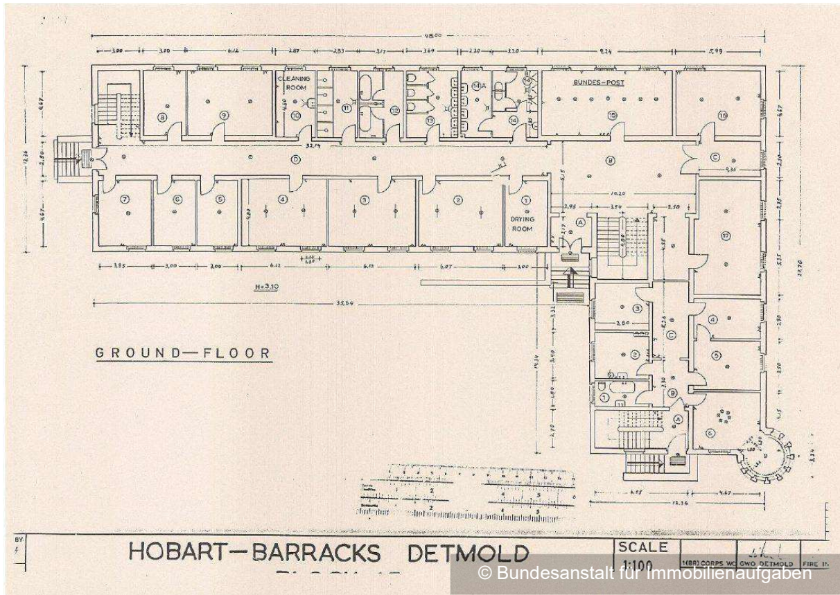
Grundriss Erdgeschoss
