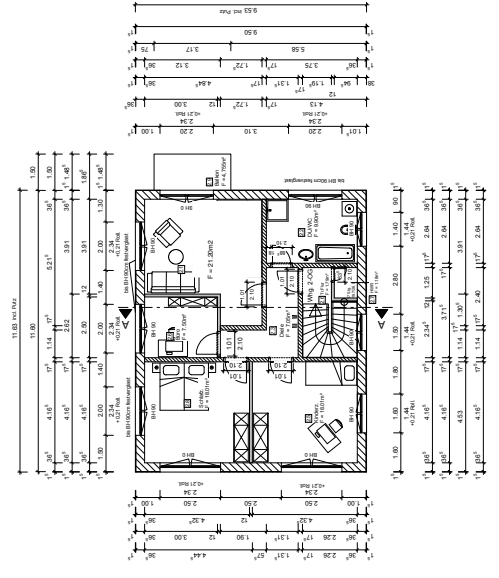
Haus 4 Grundriss Obergeschoss
