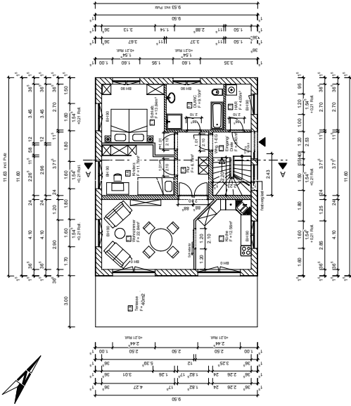
Haus 4 Grundriss Erdgeschoss
