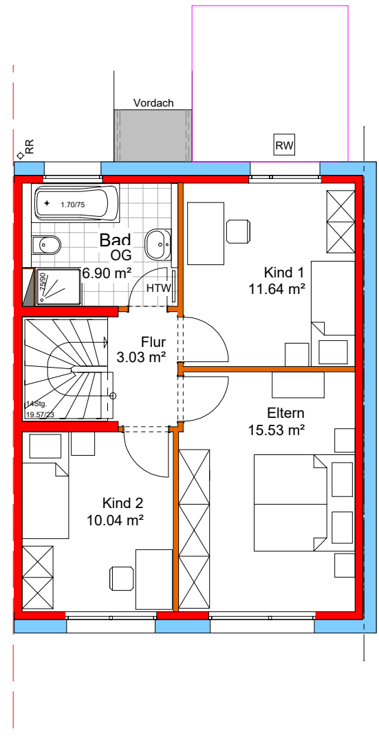
OBERGESCHOSS
