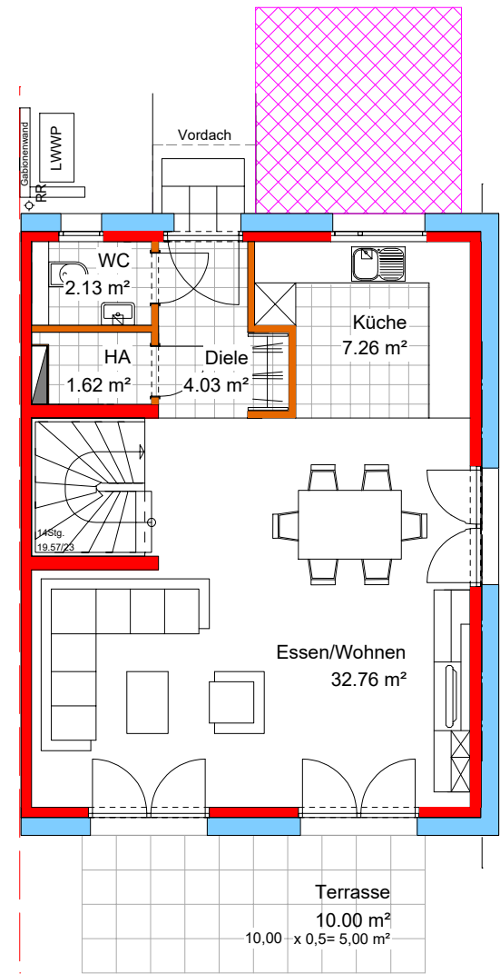
ERDGESCHOSS
