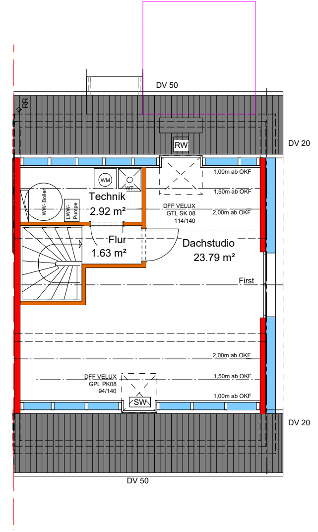
DACHGESCHOSS
