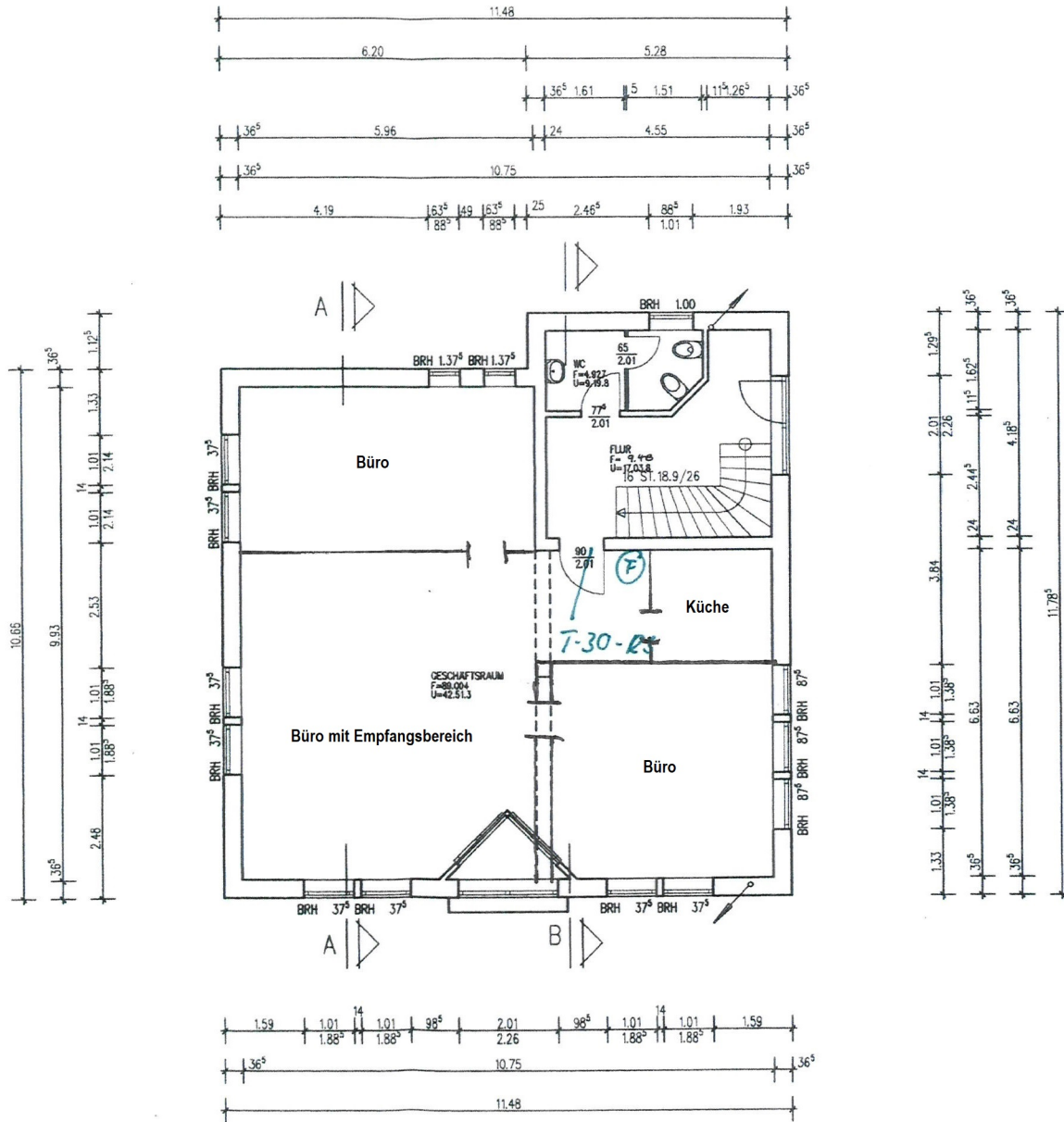
GRUNDRISS ERDGESCHOSS
