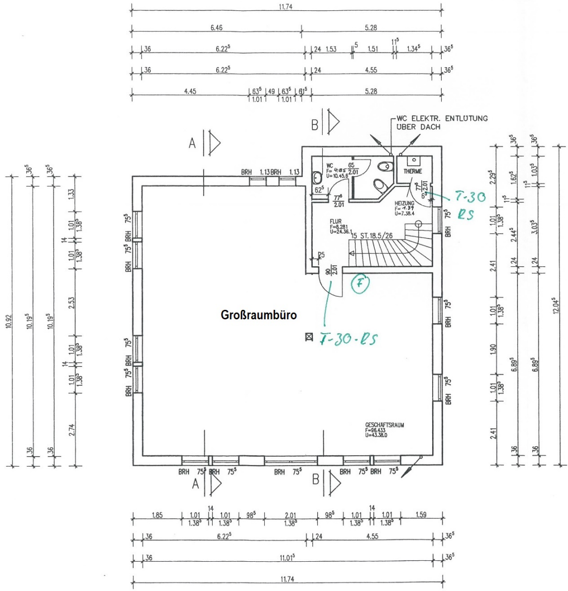
GRUNDRISS OBERGESCHOSS
