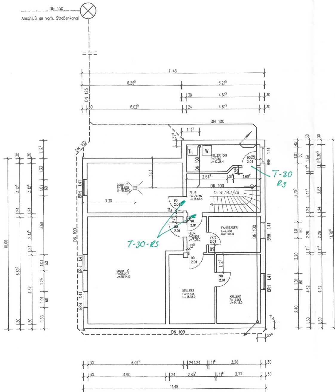
GRUNDRISS KELLERGEHOSS
