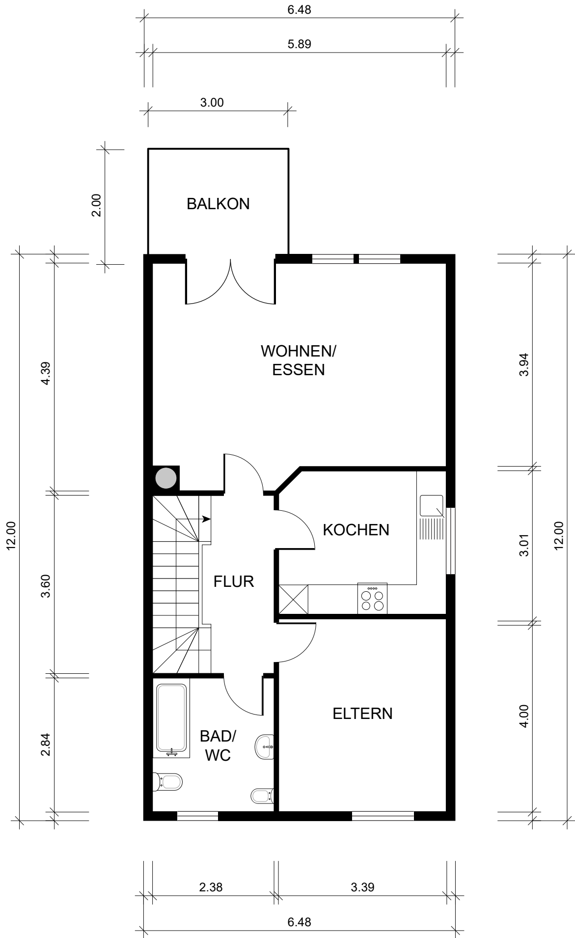
1. OBERGESCHOSS
