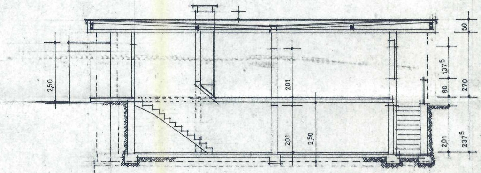
SCHNITT
