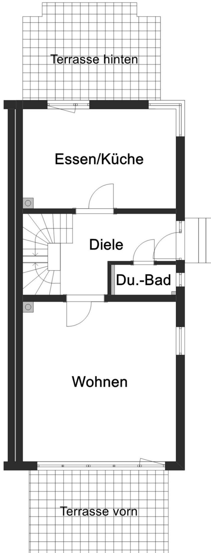
Grundriss Erdgeschoss
