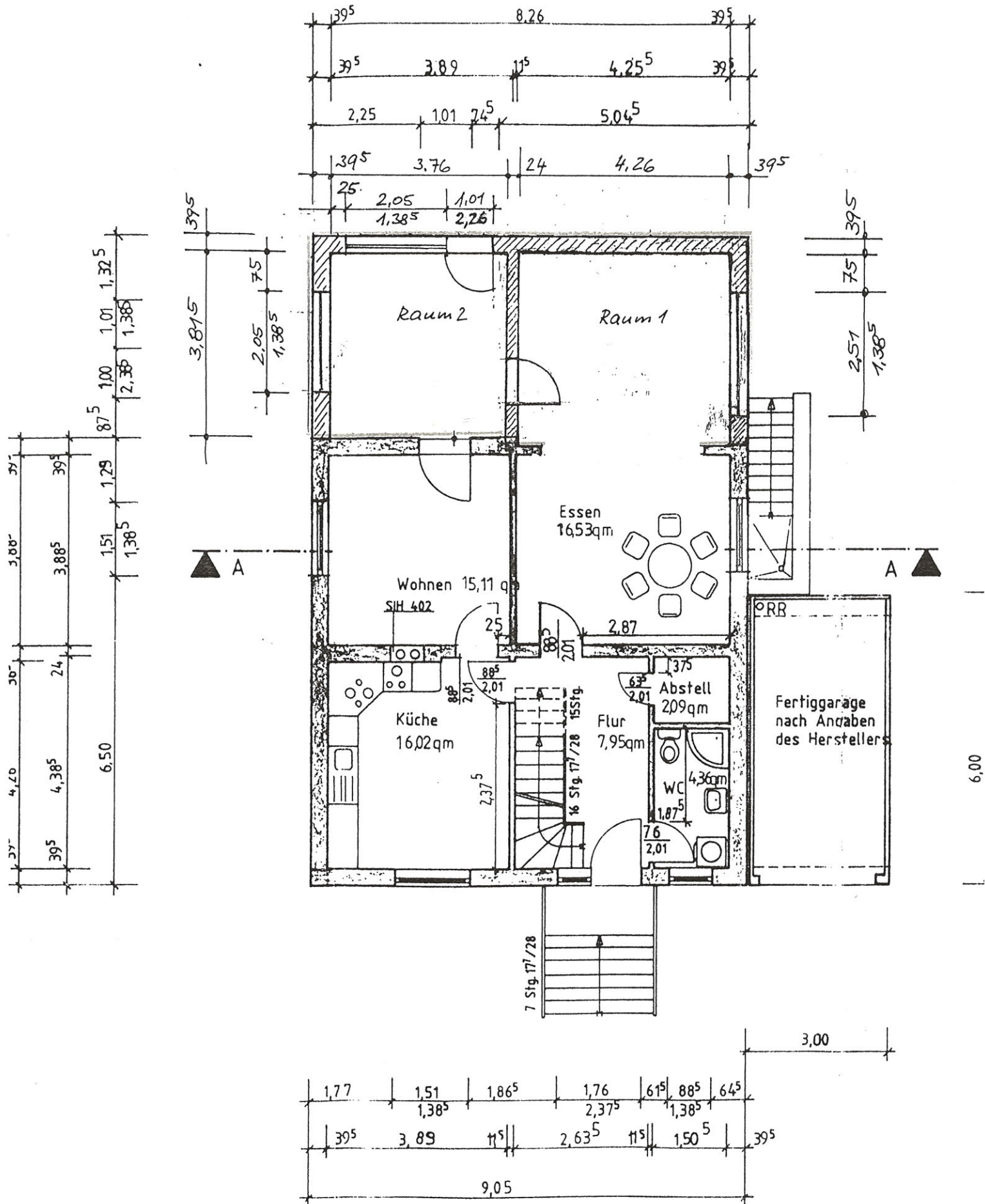
ERDGESCHOSS
