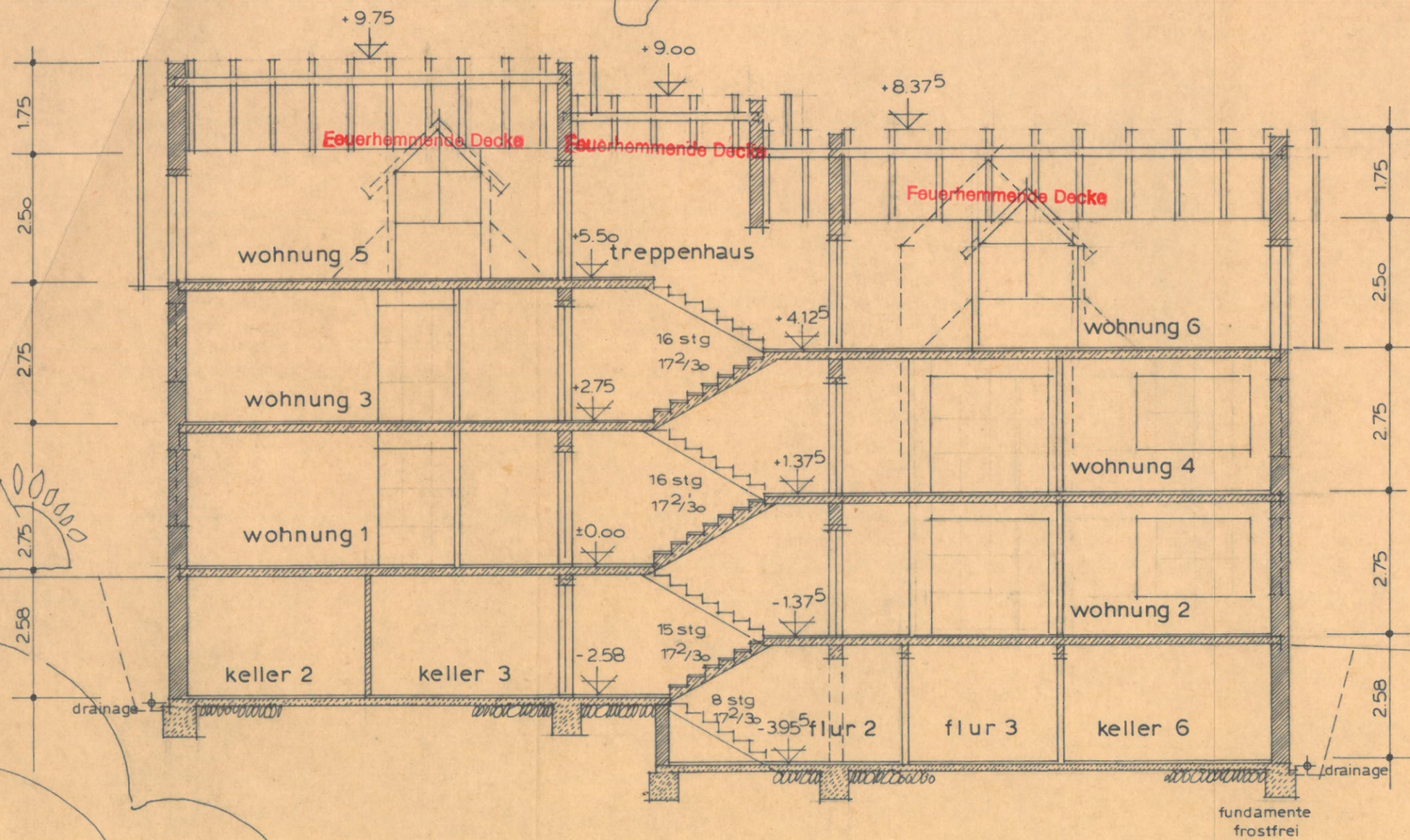
QUERSCHNITT A-B
