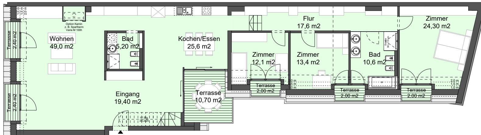
Grundriss DG
