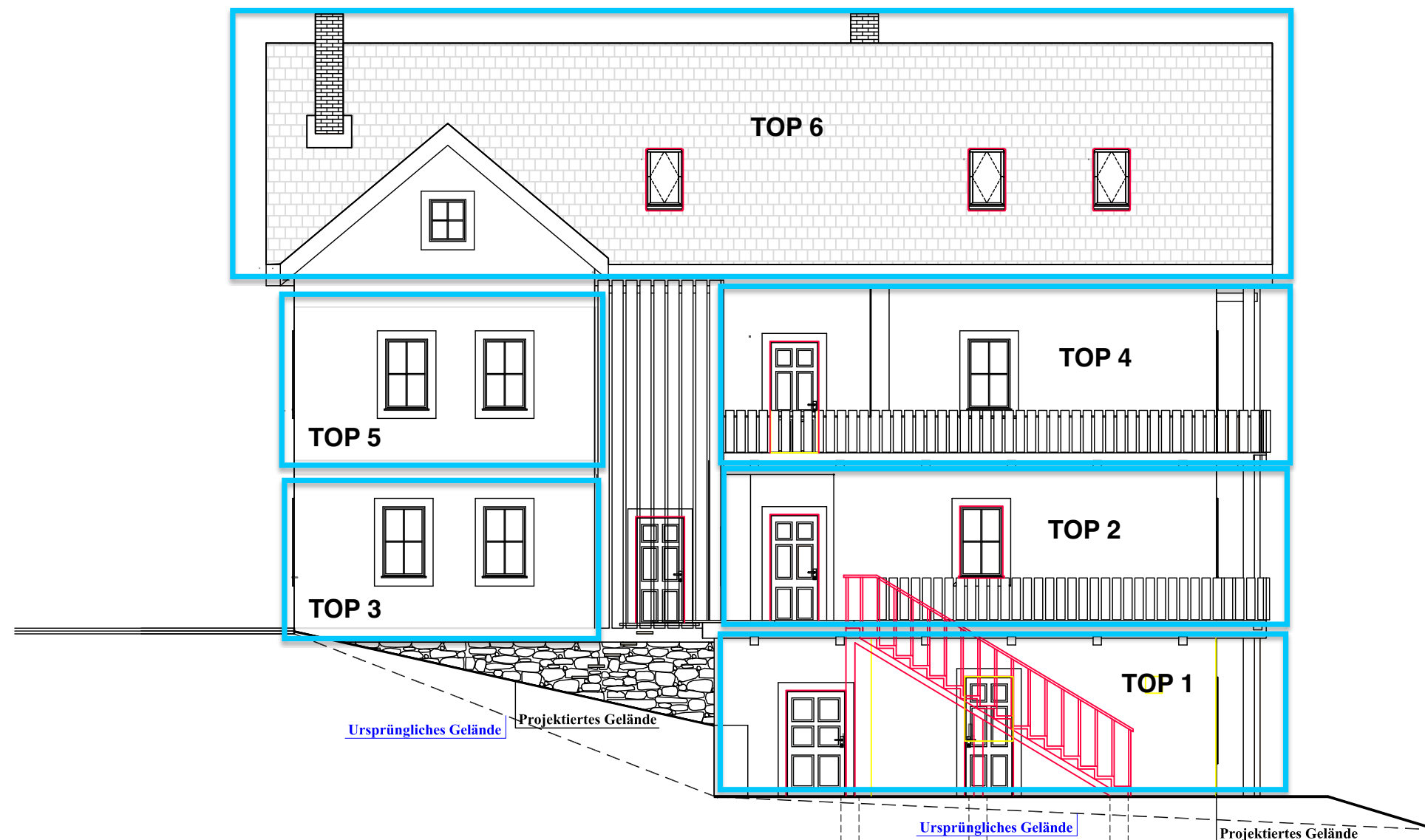
ANSICHT WESTEN
