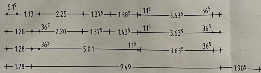
DACHGESCHOSS M. 1 : 100
