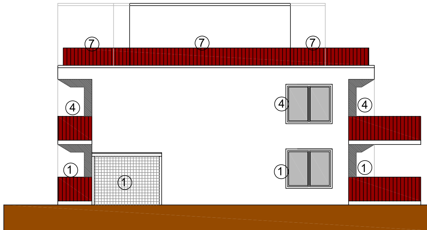
Ansicht Ost
