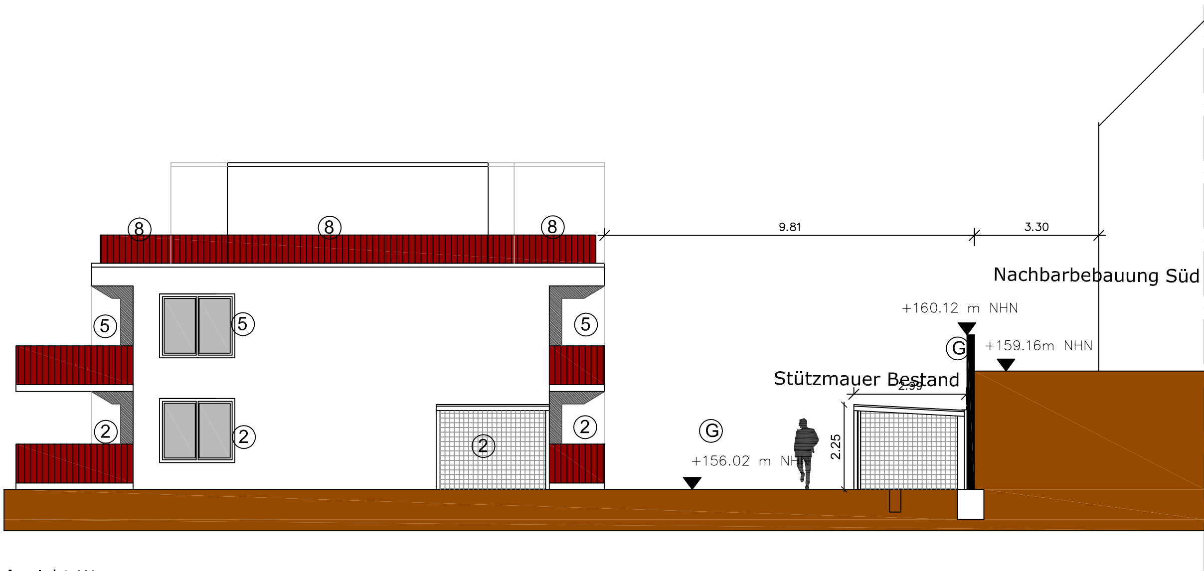
Ansicht West
