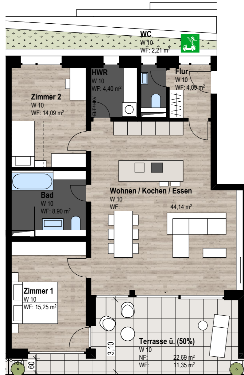
W 10 M1:100
