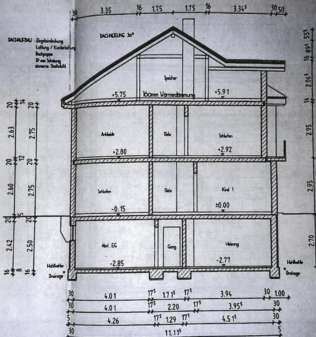
SCHNITT A / A
