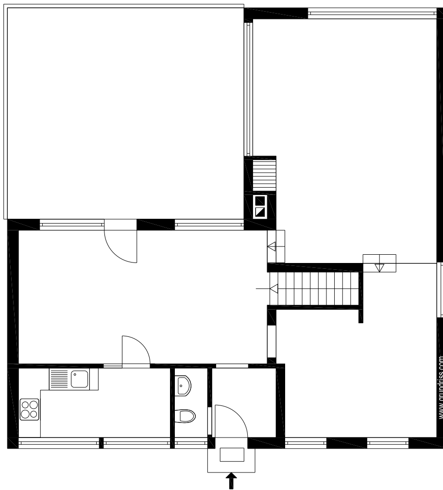
Erdgeschoss
