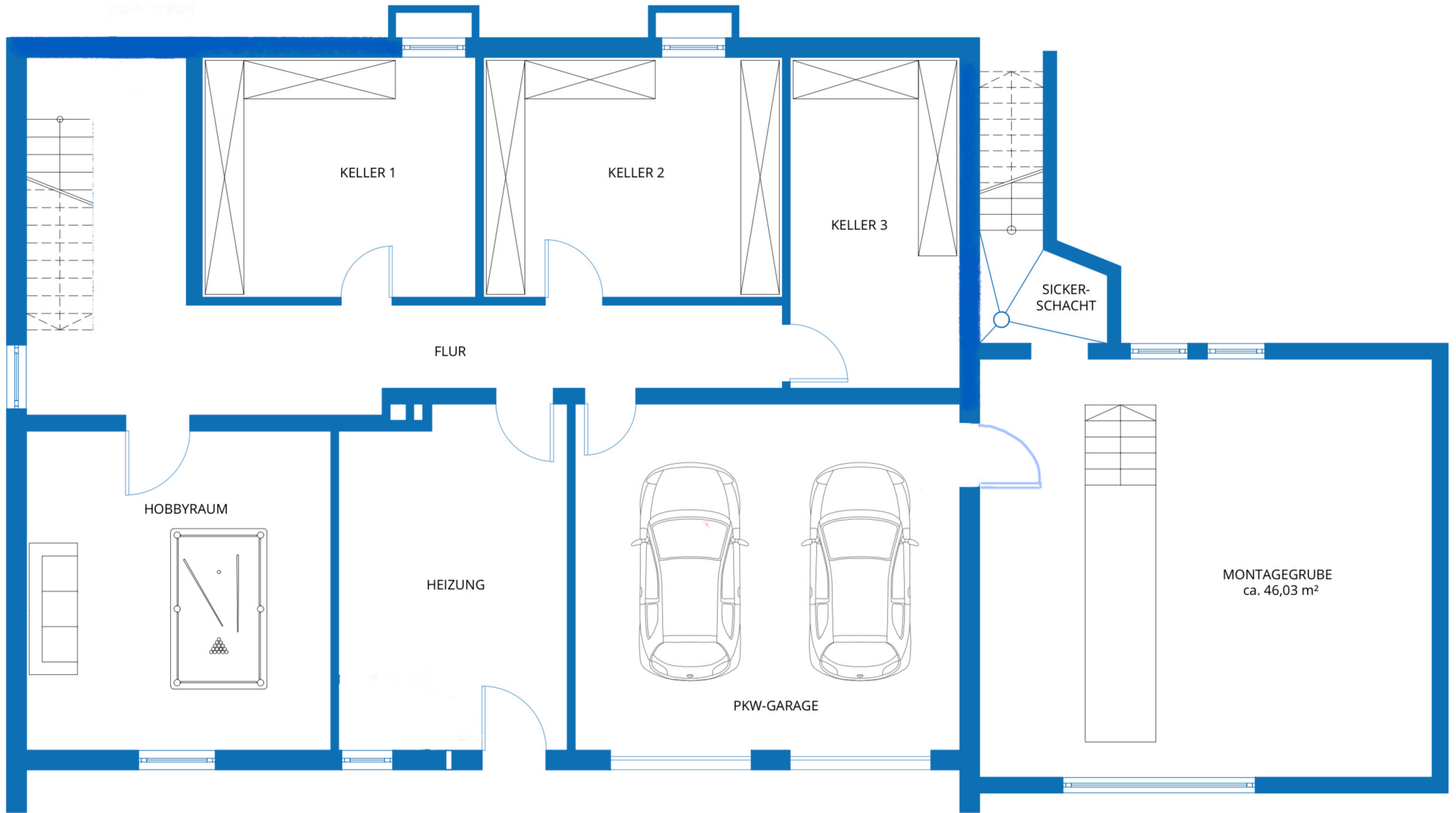
Kellergeschoss
