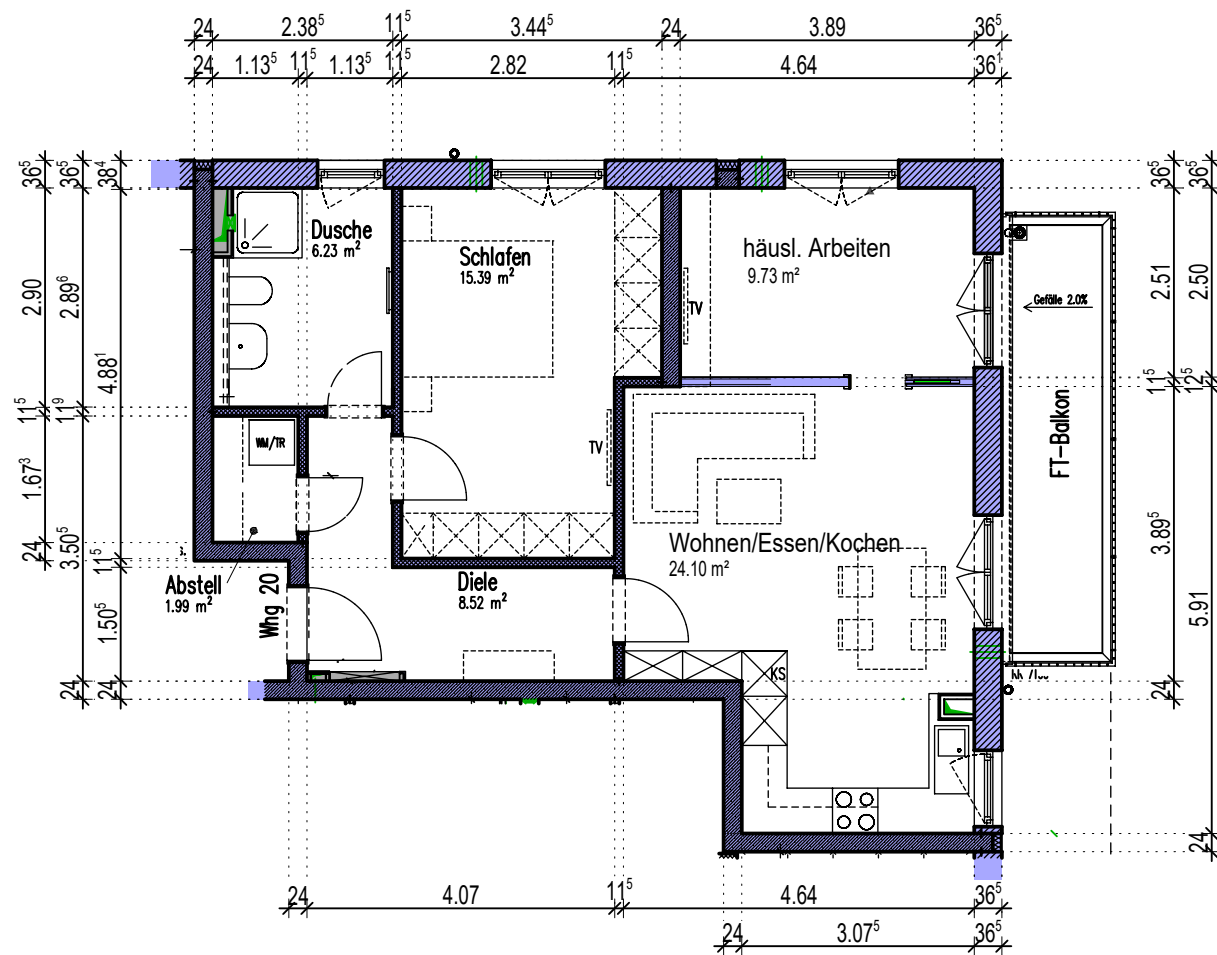
Olching Pfarrstraße - Wohnung 20 M1:100
