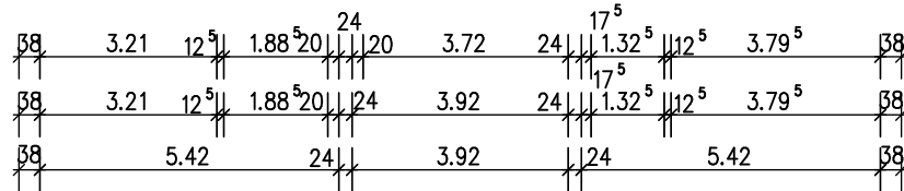
4.OG Haus I Wohnungen 17-18 M1:100
