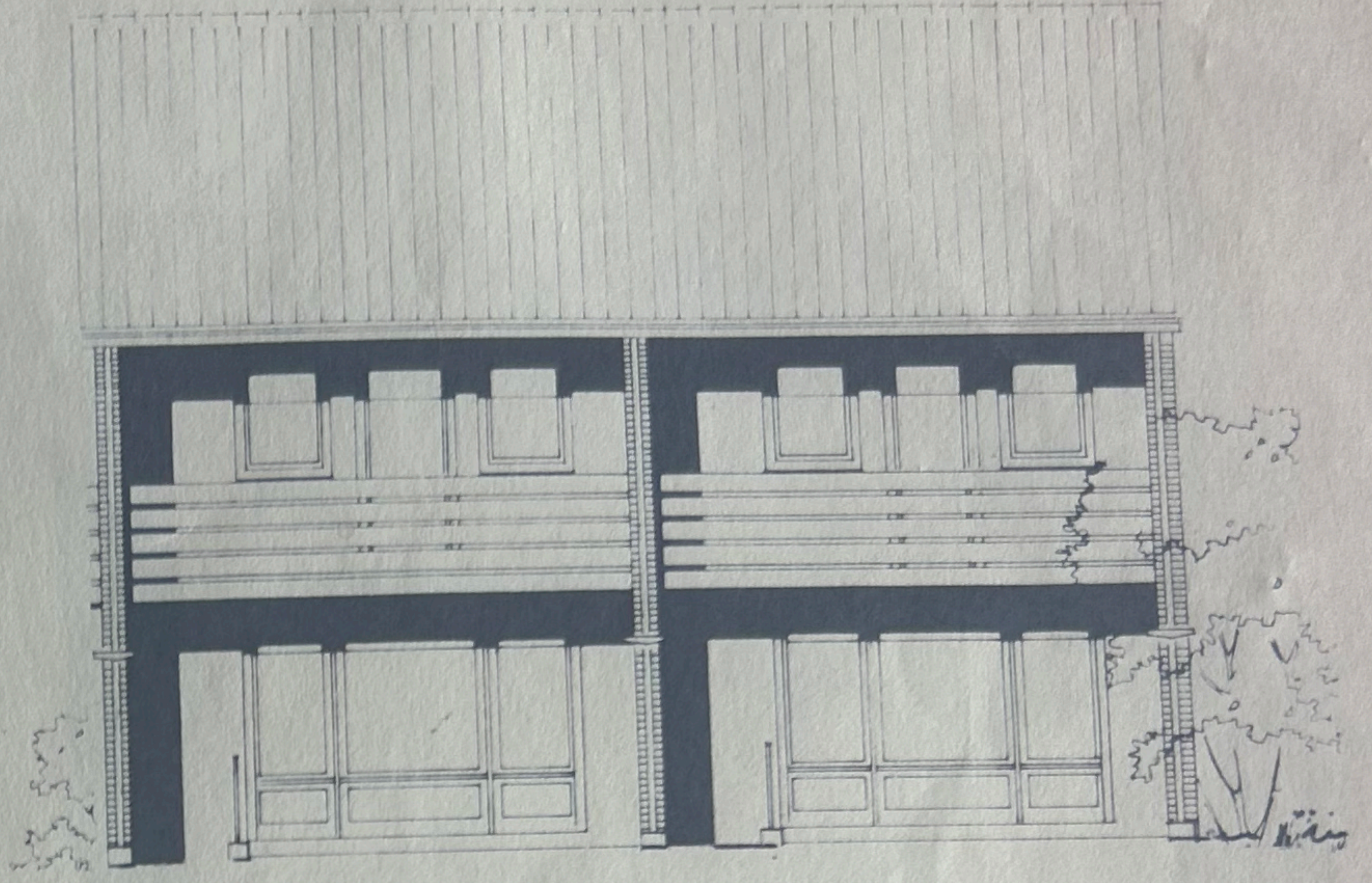
GARTENANSICHT
