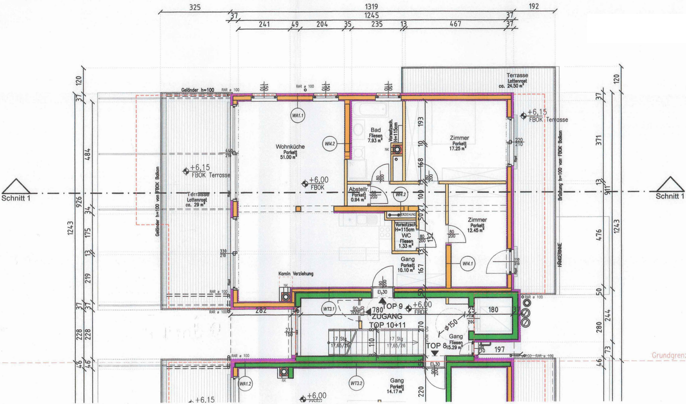
1. Dachgeschoss
