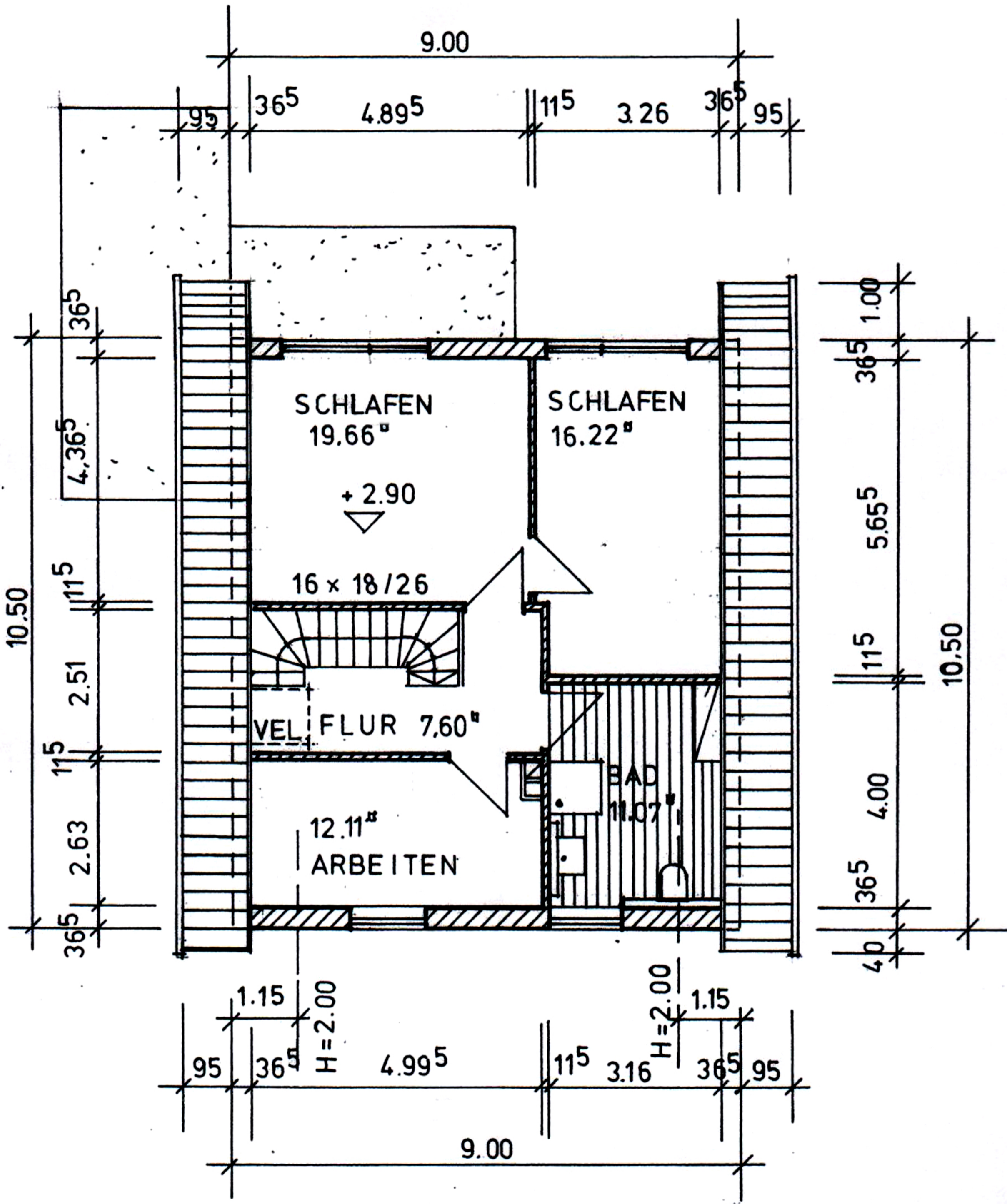
1. OBERGESCHOSS
