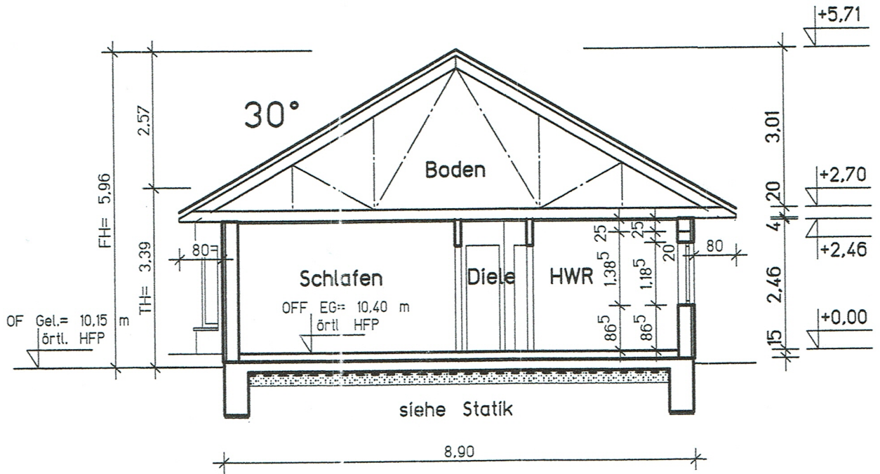
Schnitt A-A
