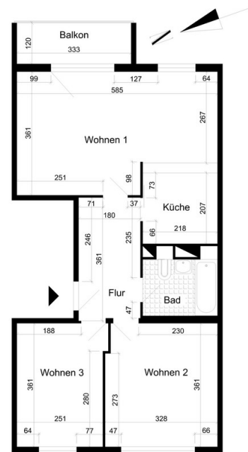
Grundriss
