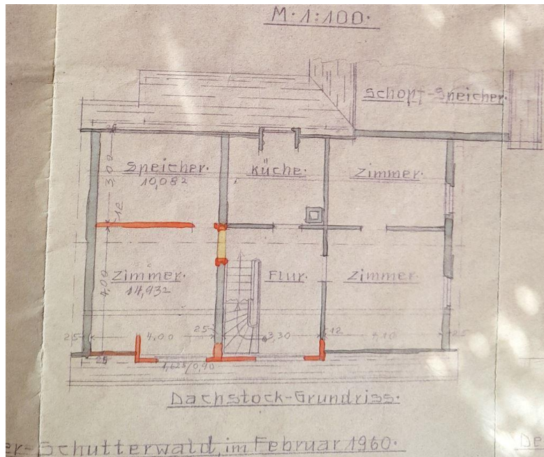
Grundrisse DG
