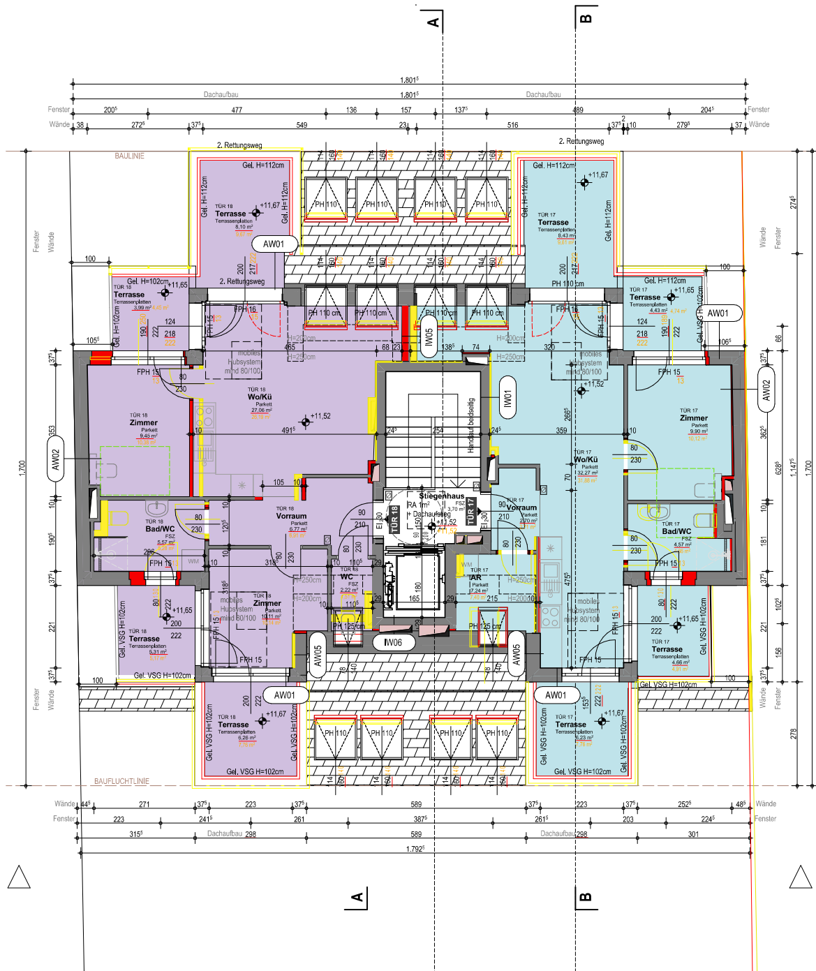
2. DACHGESCHOSS
