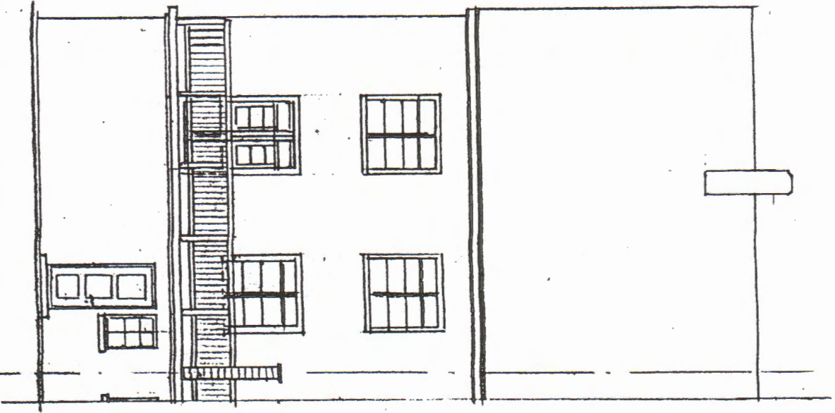
Rück-(Ost-) Ansicht
