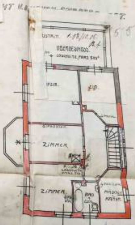
OBERGESCHOSS:
