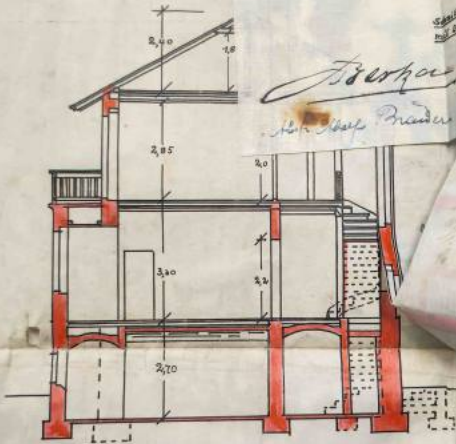
SCHNITT A-B.
