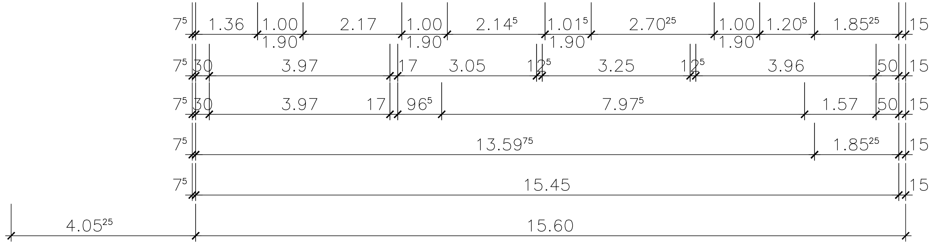
OBERGESCHOSS BESTAND / NEUPLANUNG M 1 : 50
