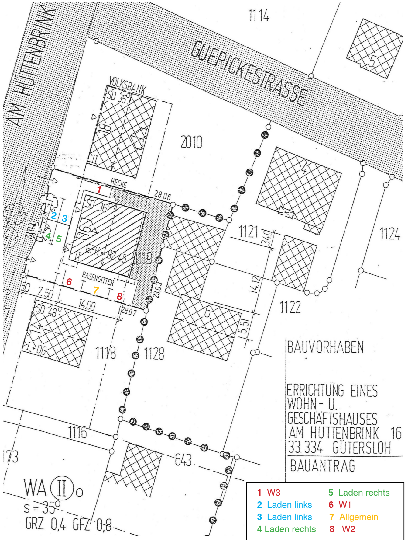
Lageplan
