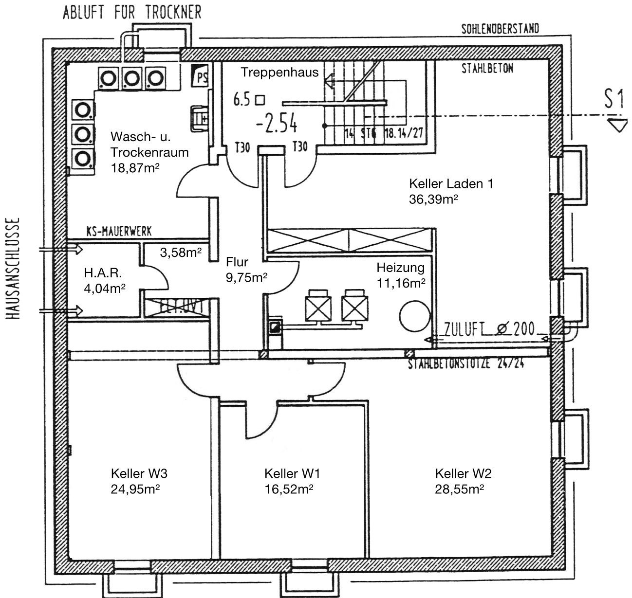
Kellergeschoss
