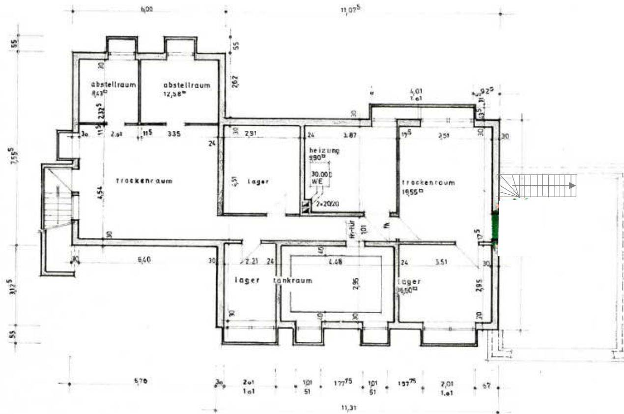
kellergeschoss
