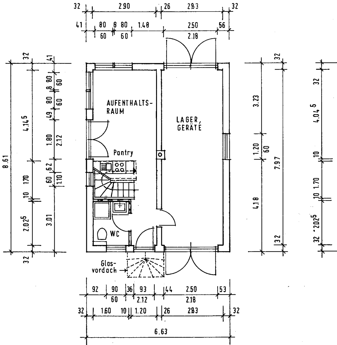
ERDGESCHOSS
