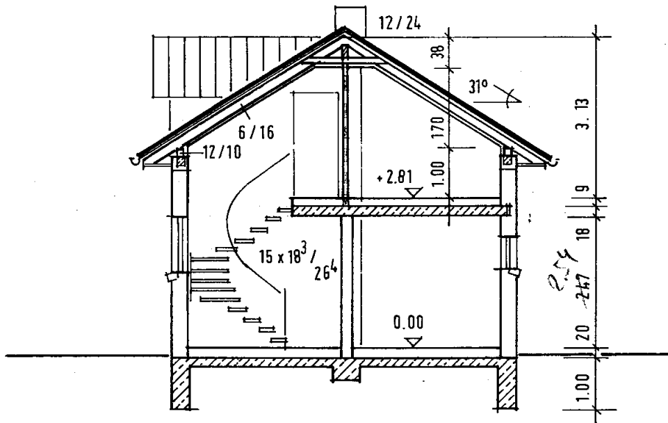
SCHNITT
