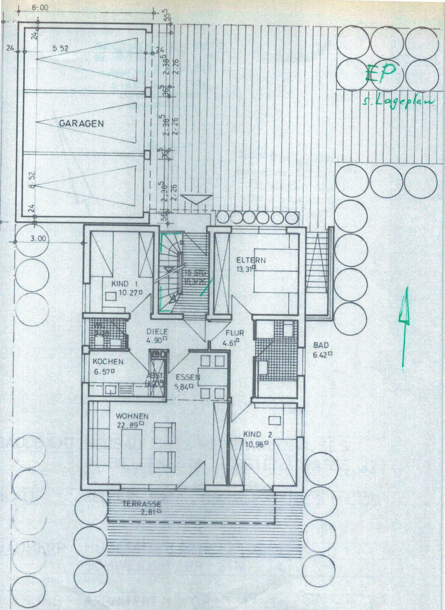
ERDGESCHOSS (WOHNFLÄCHE 90,60 qm)
