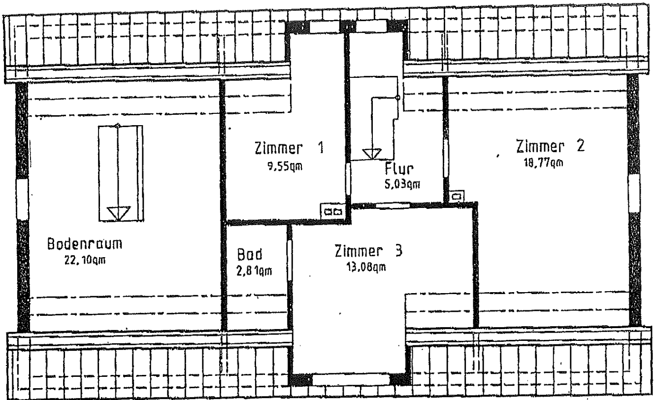
Dachgeschoss, M. 1:100
