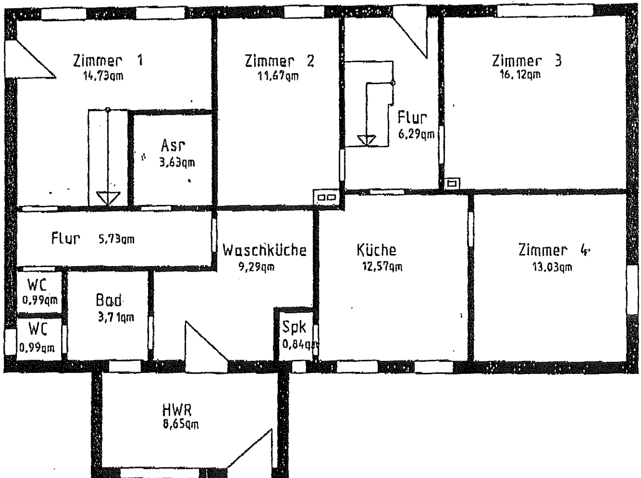
Erdgeschoss, M. 1:100
