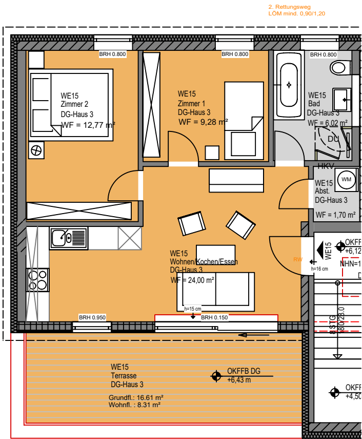
Dachgeschoss WE15
