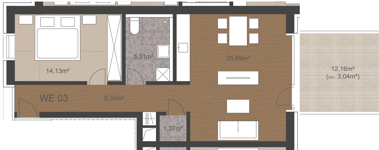
Baufeld 4 Punkthäuser Erdgeschoss WE 03 - 59,05m 2
