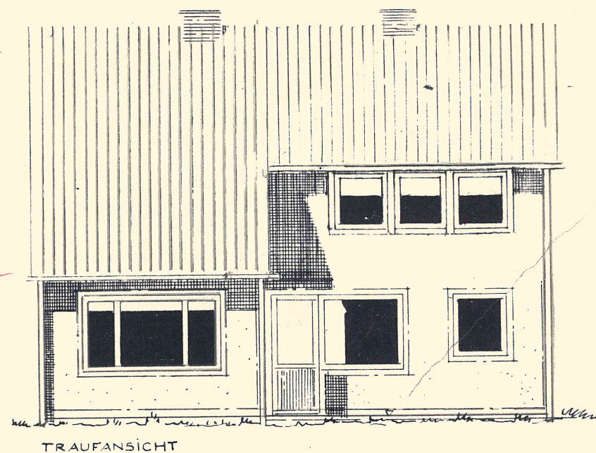
TRAUFANSICHT
