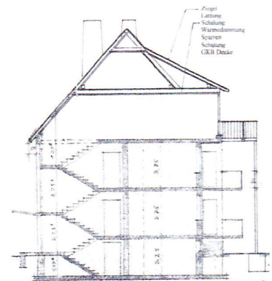
Schnitt
