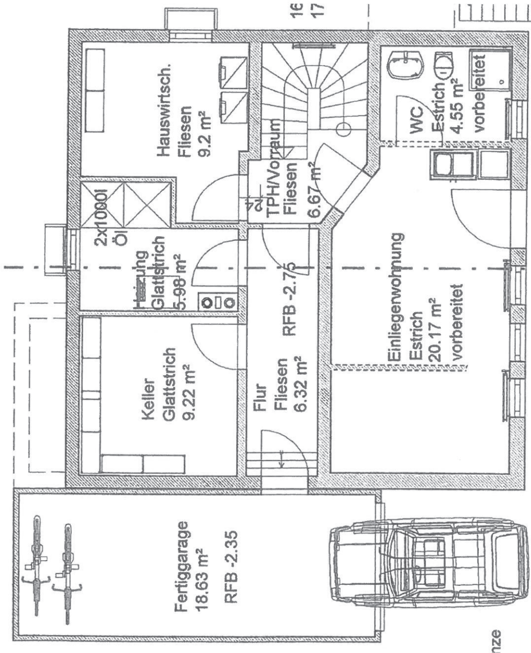
Grundriss Untergeschoss
