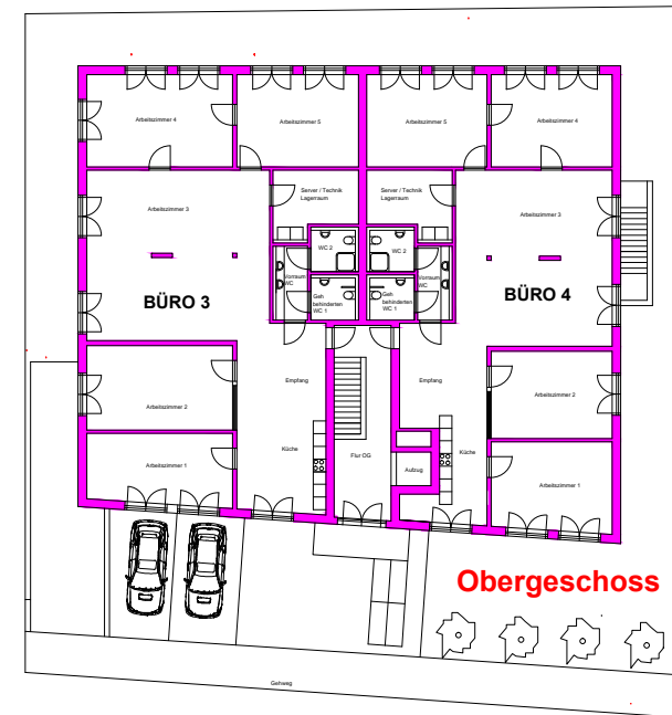
Obergeschoss OG
