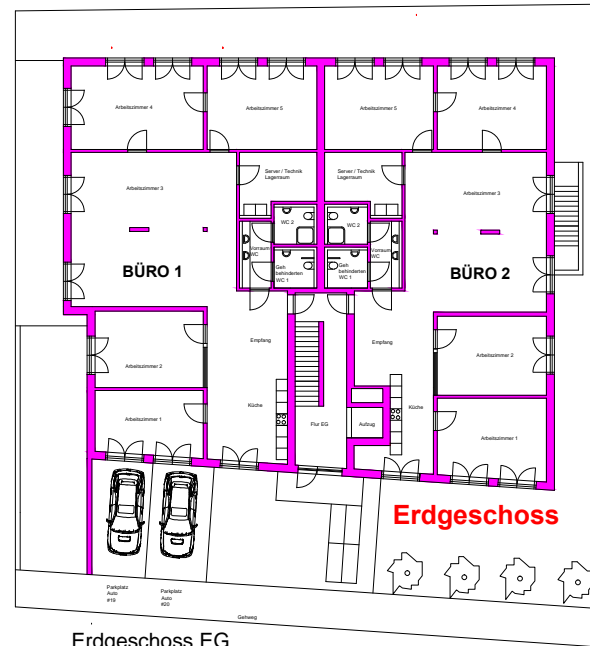
Erdgeschoss EG
