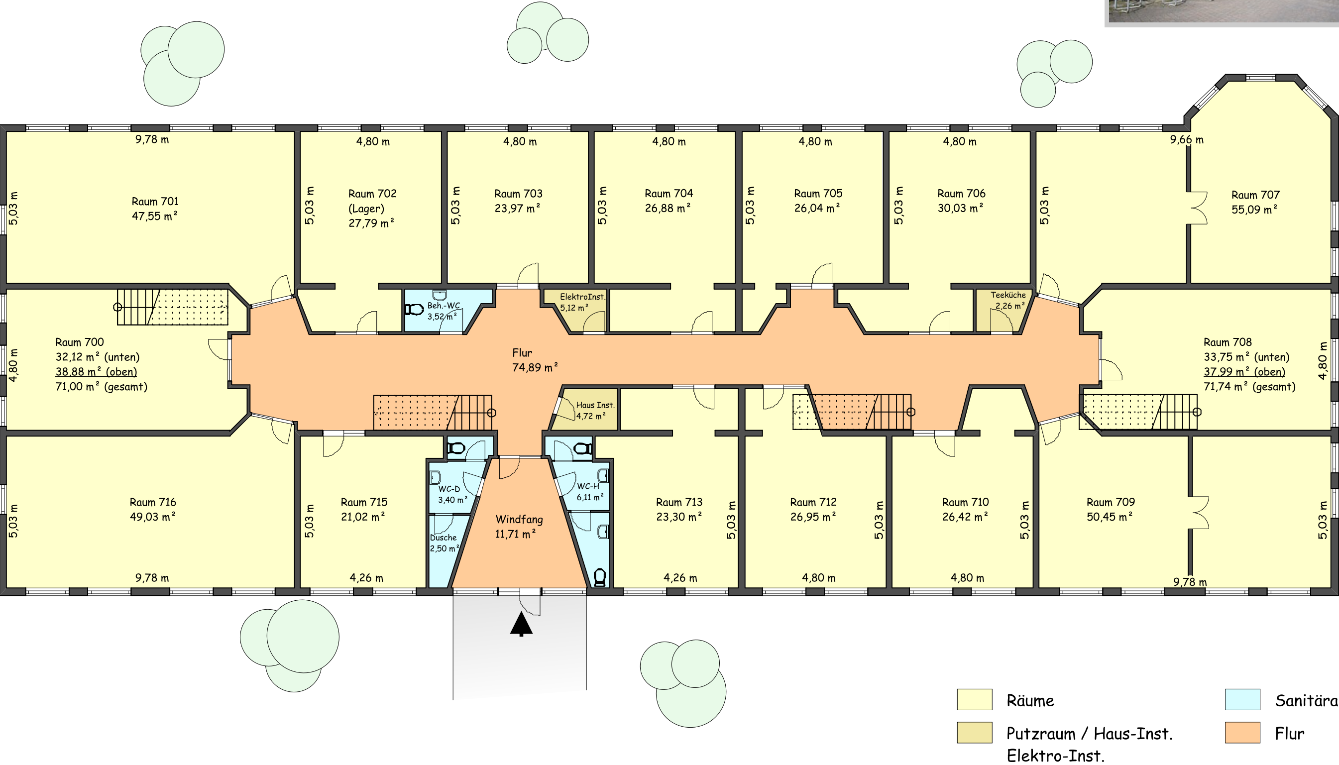
Erdgeschoss Zeichnung ohne Maßstab
