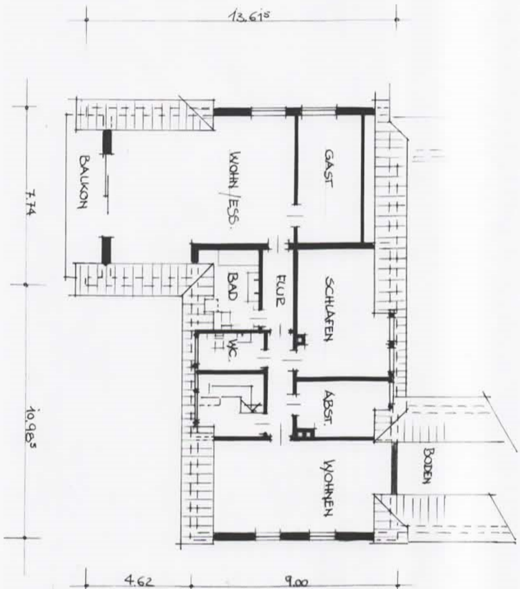
DACHGESCHOSS H. 1:100
