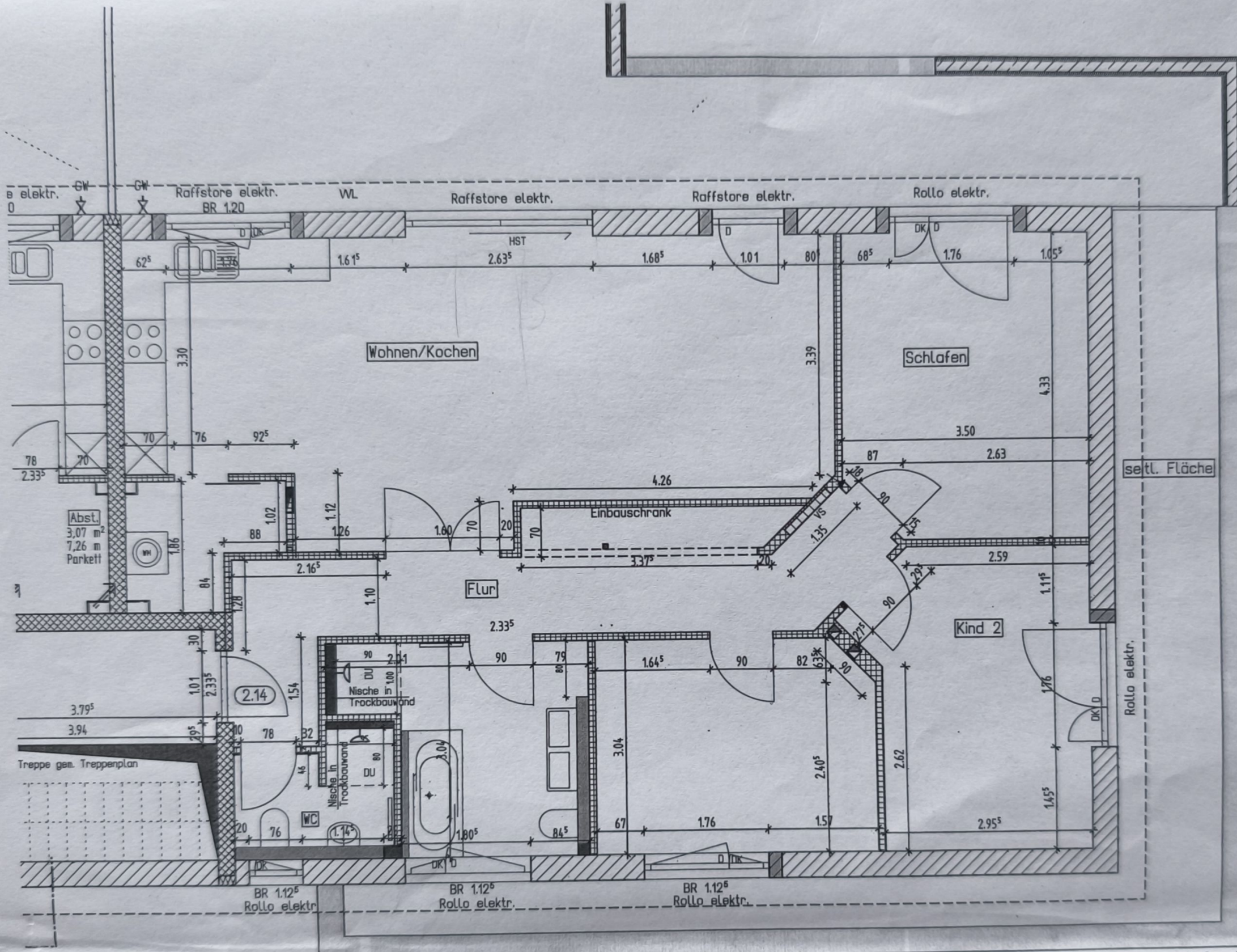
Vermaßter Grundrissplan Wohnung 2.14 WICHTIG: Bei den angegebenen Maßen handelt es sich um Rohbaumaße! Diese müssen vor Ort nachgemessen werden!! M= 1:50 4.11.2019
