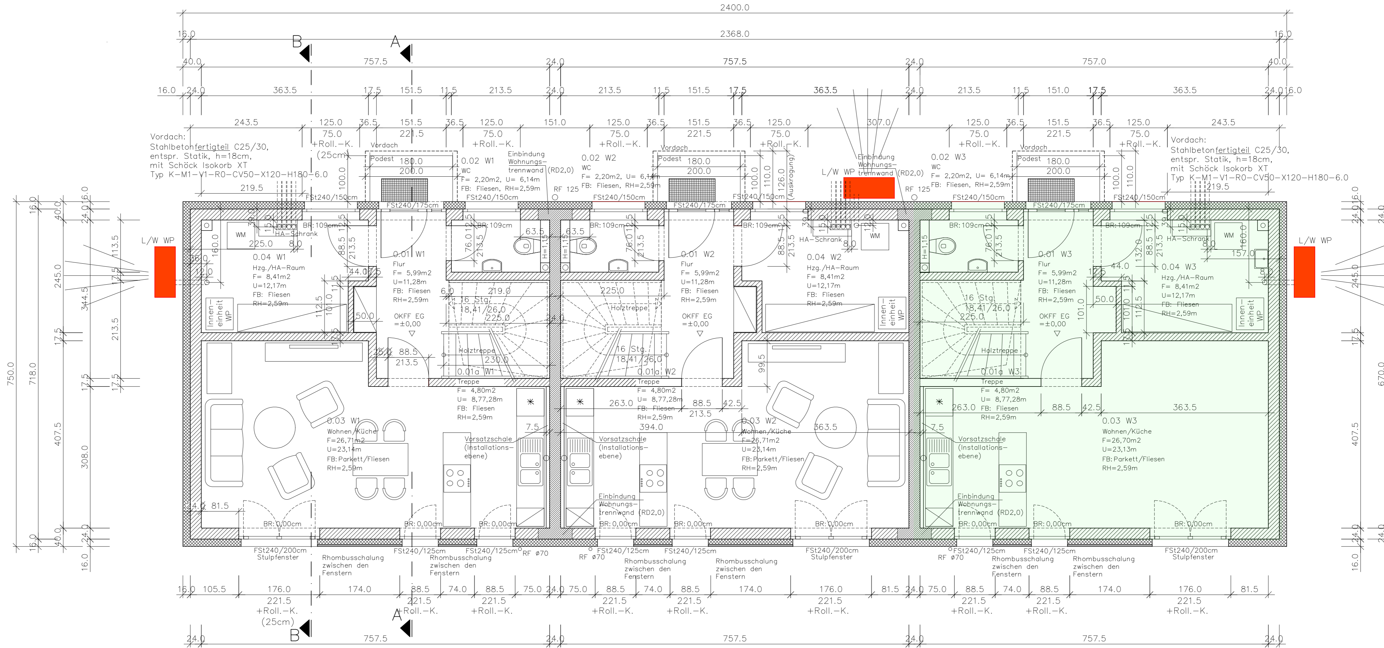
Grundriss Erdgeschoss
