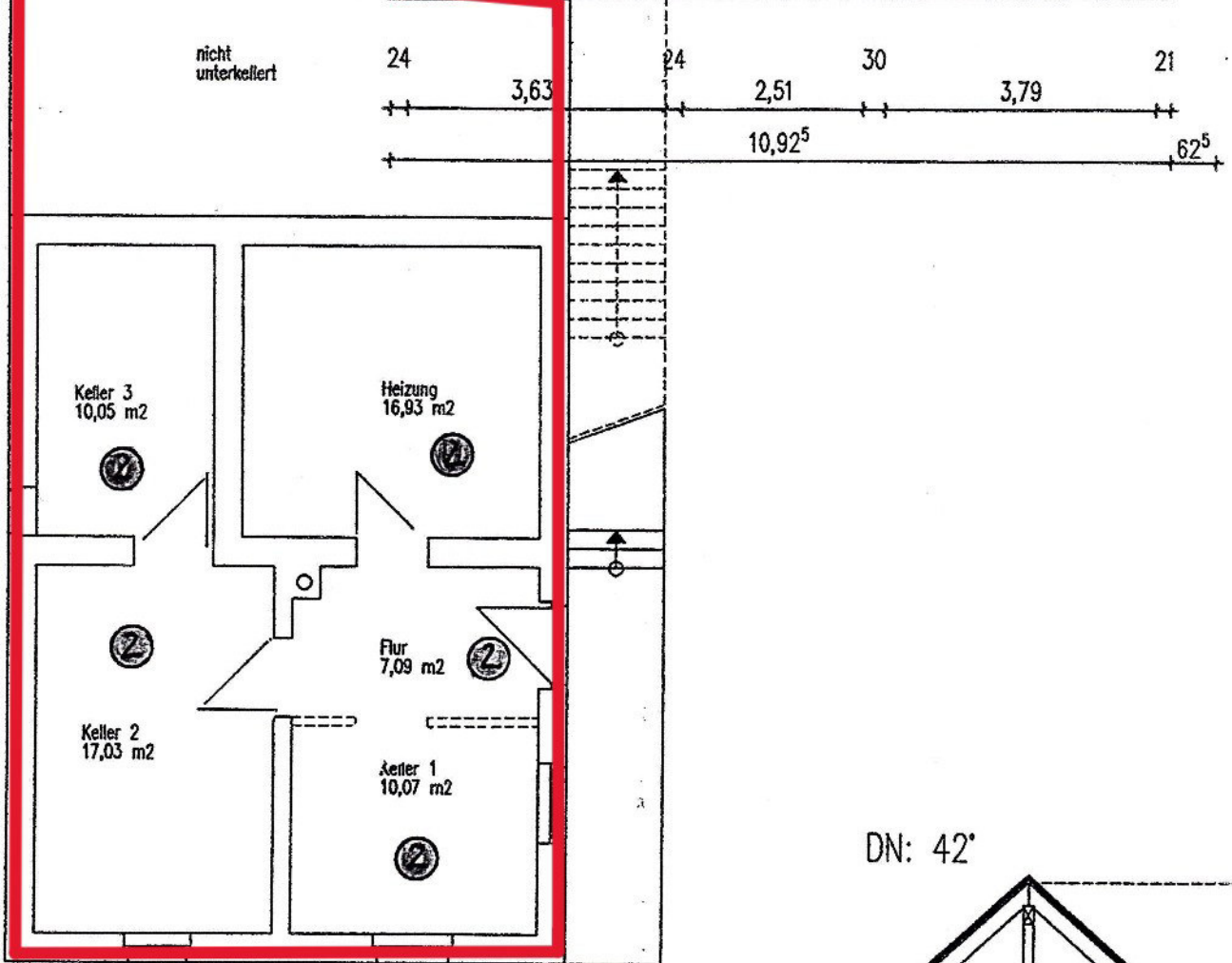
Wohnung Kellergeschoß
