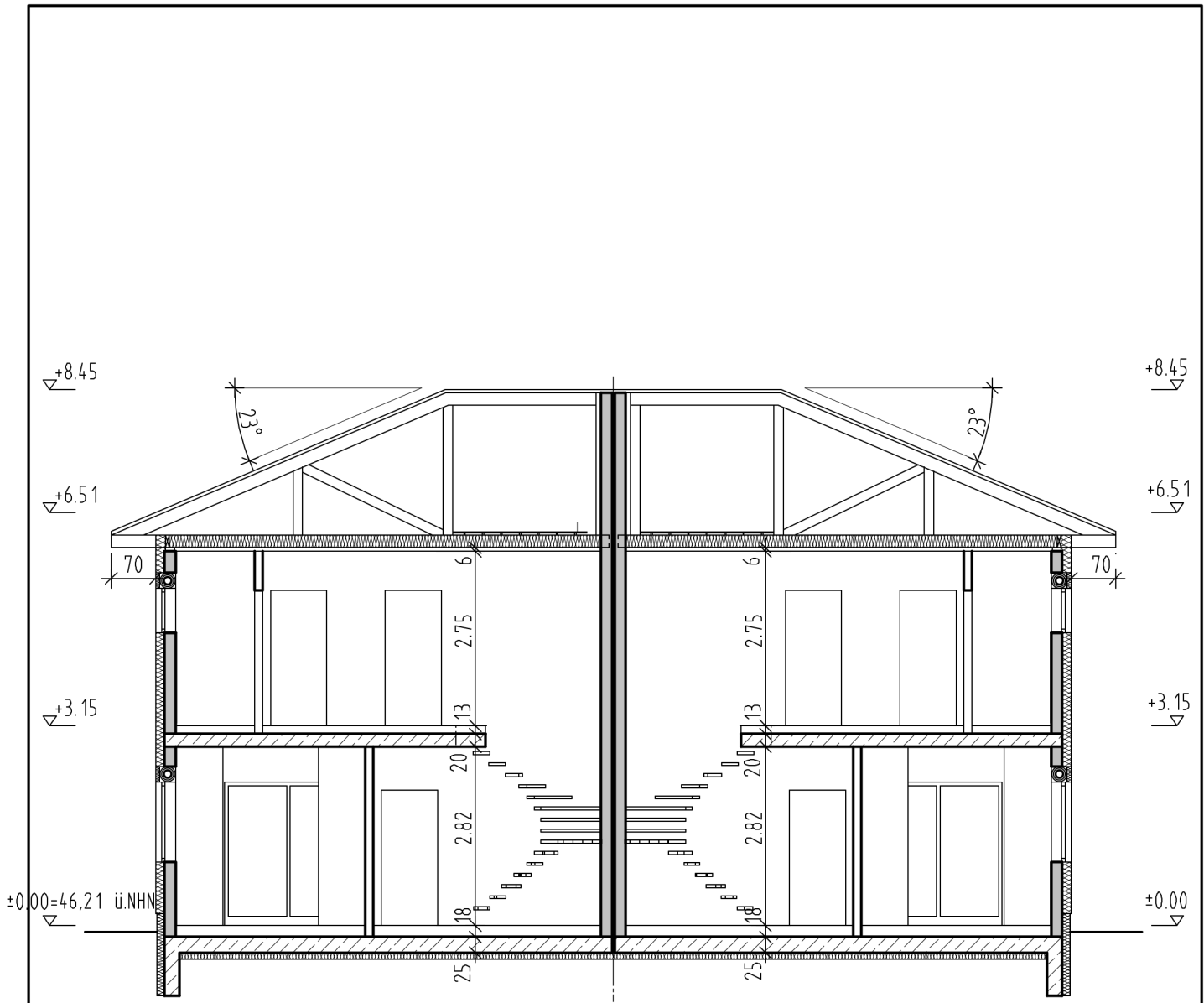
SCHNITT A-A
