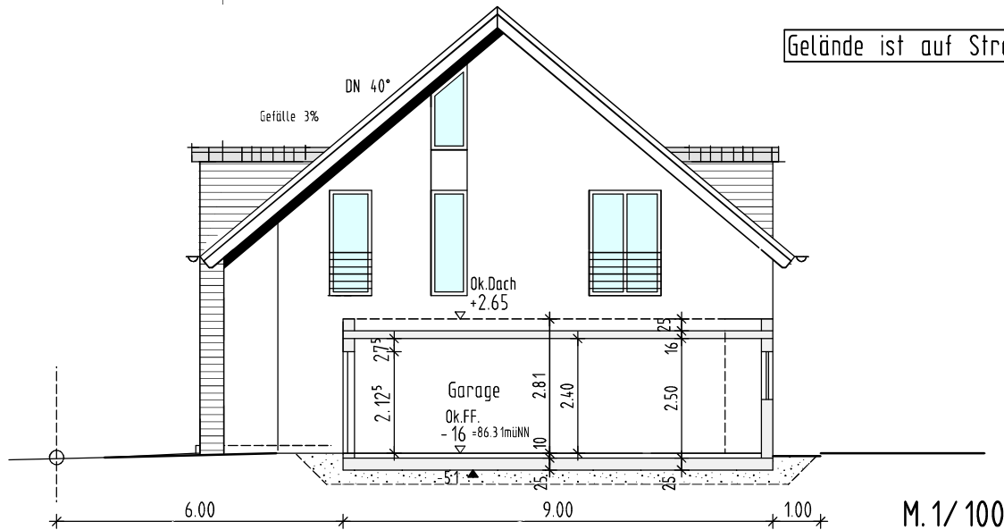
ANSICHT GARTEN M. 1/100
