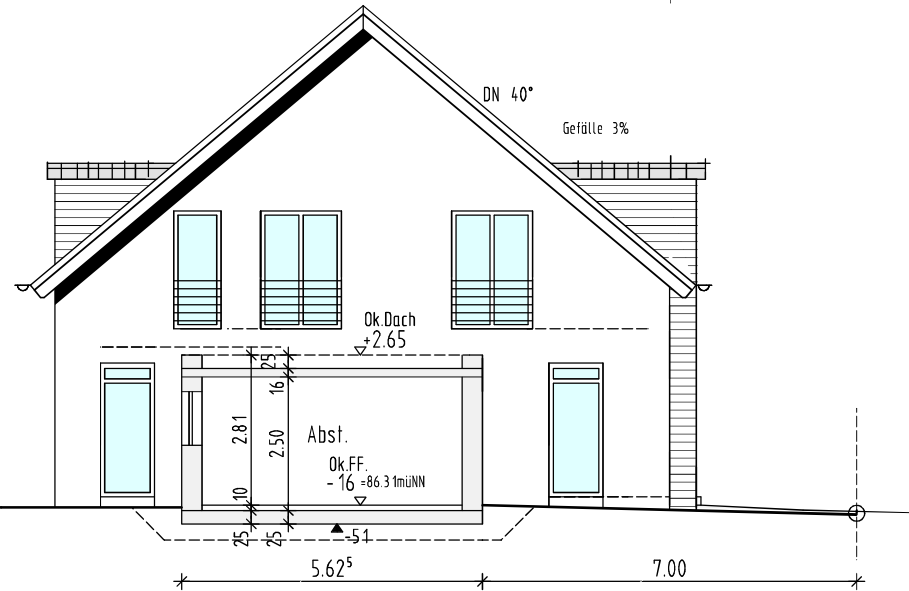
ANSICHT SEITE/ SCHNITT ABST. M. 1/100
