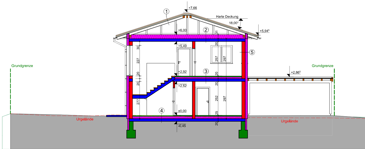
Schnitt A - A
