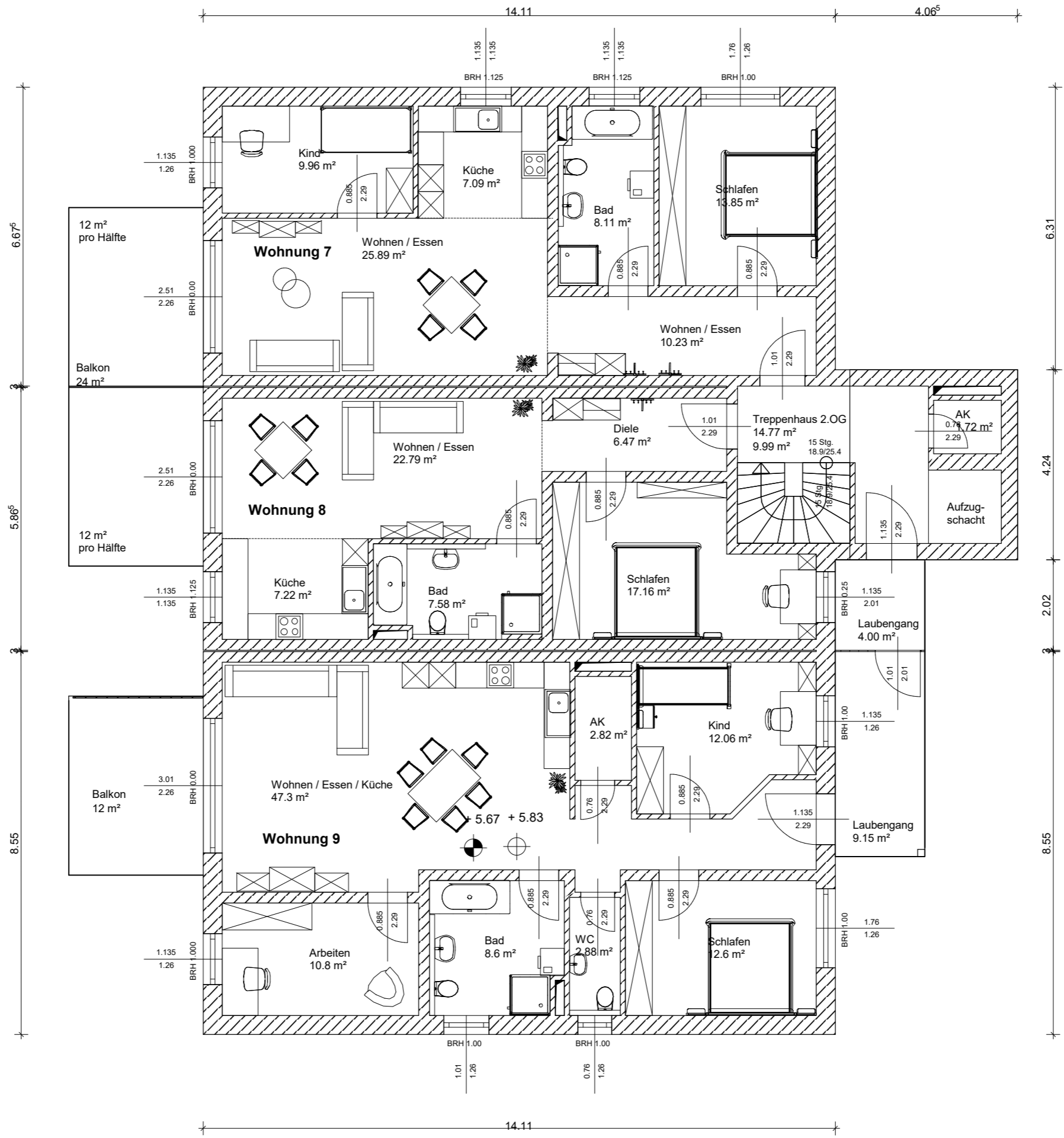
Grundriss 2. Obergeschoss
